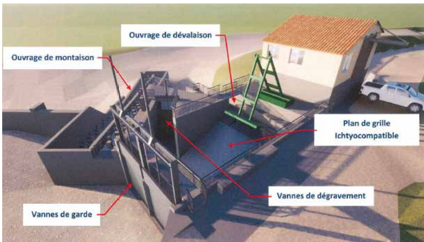
Figure 33 - Illustration 3D de la nouvelle prise d'eau
